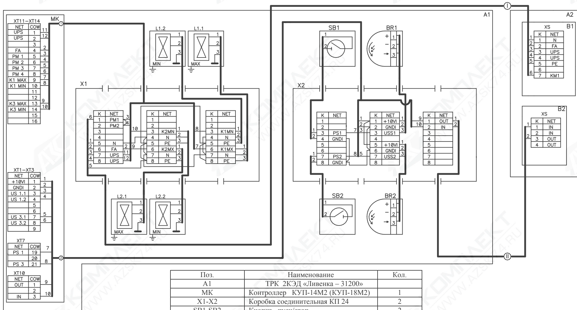
Рисунок В.5 - Схема электрическая обшая ТРК 2КЭД «Ливенка-31200»
