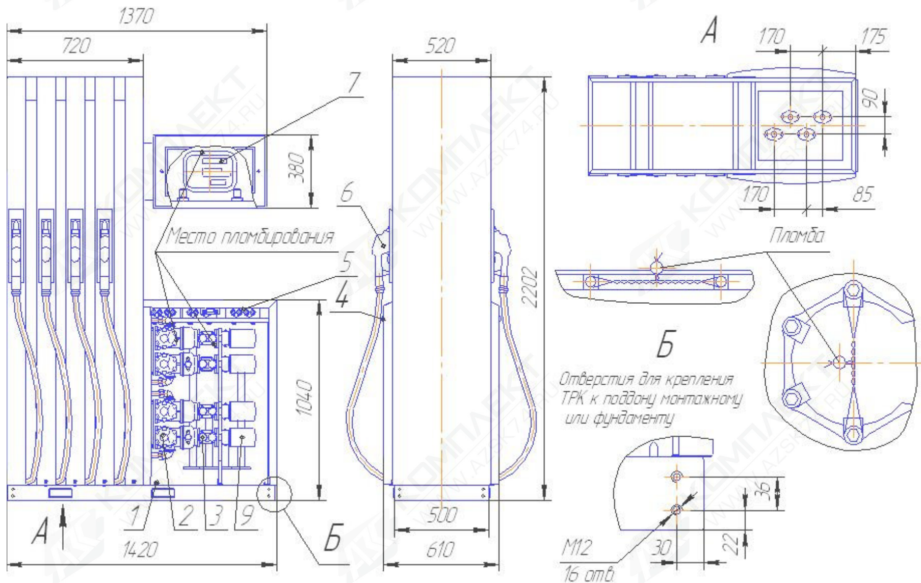
Рисунок А.1 – ТРК «Ливенка 2КСД «Ливенка-34800».
