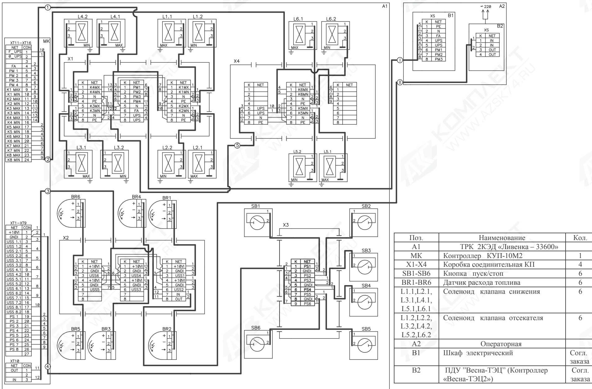
Рисунок Б.3 - Схема электрическая общая ТРК 2КЭД «Ливенка-33600»
