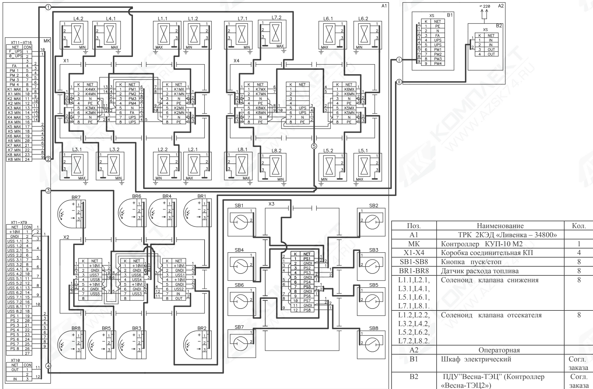
Рисунок В.2 - Схема электрическая общая ТРК 2КЭД «Ливенка-34800»
