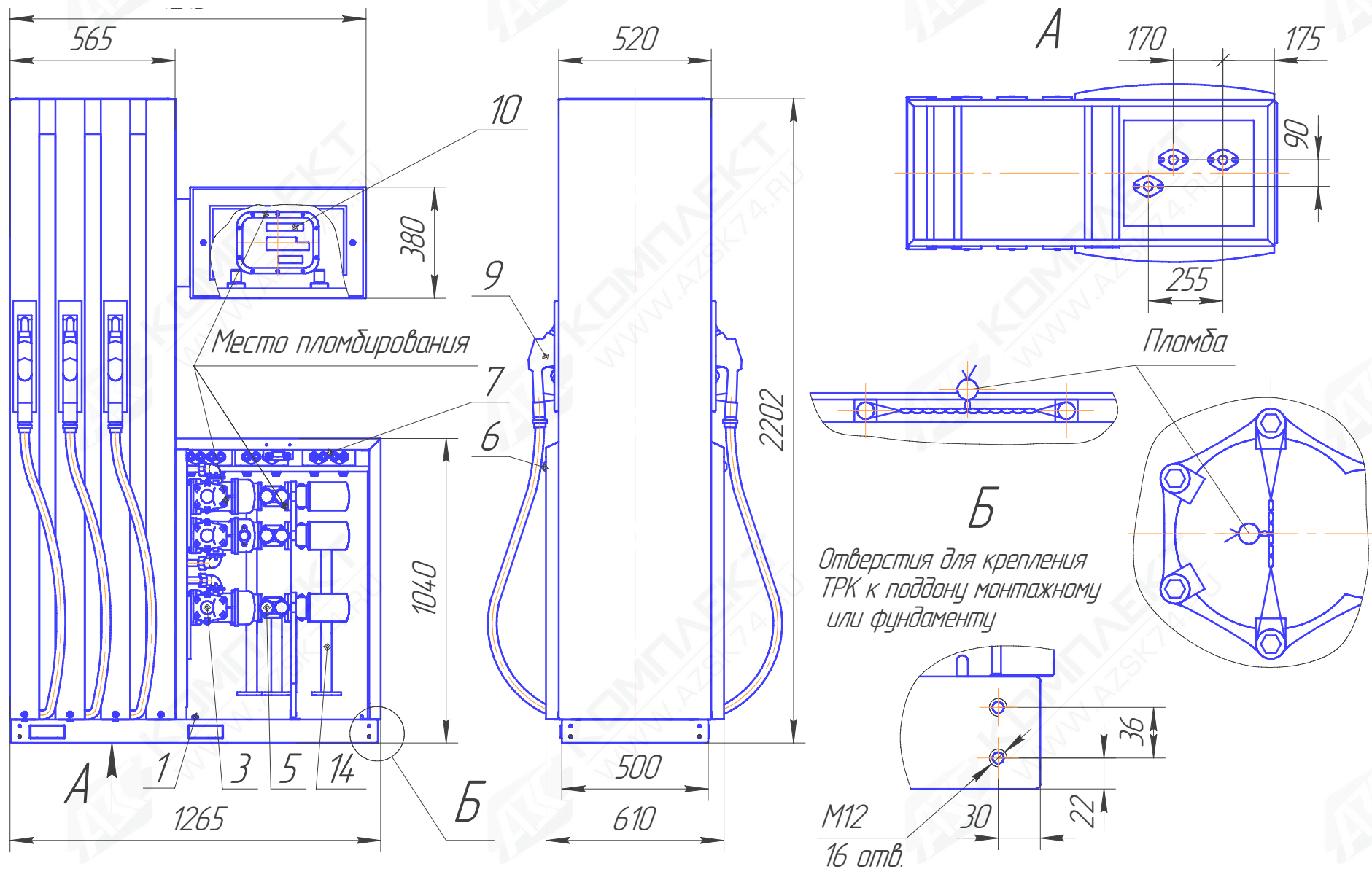
Рисунок А.2 – ТРК 2КСД «Ливенка-33600». Габаритные и присоединительные размеры.
