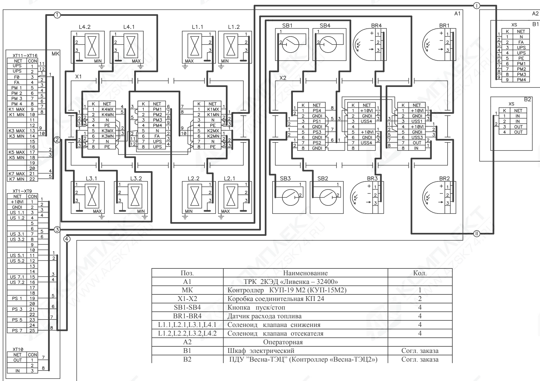
Рисунок Б-4 - Схема электрическая общая ТРК 2КЭД «Ливенка-32400»
