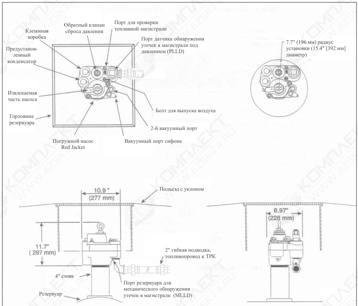
Рисунок 1. Компоненты и размеры головы насоса Red Jacket.
