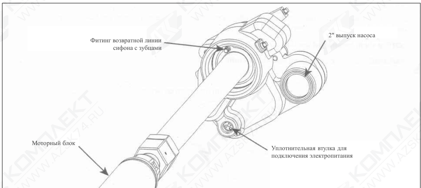
Рисунок 2. Основные компоненты насоса.
